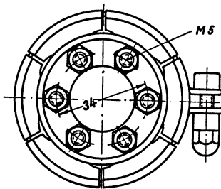
Anschlußkappe Lager-Nr. 30361
