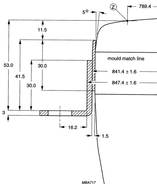
Fig.8 Lug position.
