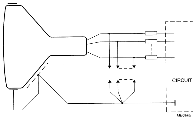
Fig.1 Flashover protection circuit.
