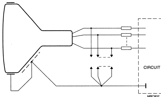
Fig.24 Flashover protection circuit.
