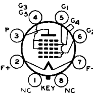
G-7Z
