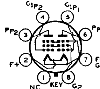
G-8C
