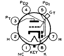
G-7V
