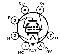
G-7AC
