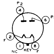
G-5T
