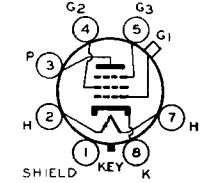
G-7R (6J7-G)
