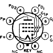
G-7AD
