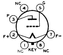
G-5S
