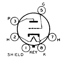
G-6Q
