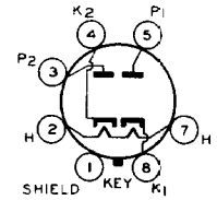
G-7Q
