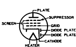
DUPLEX-DIODE PENTODE
