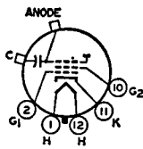
12N ANODE = G_3 + CL
